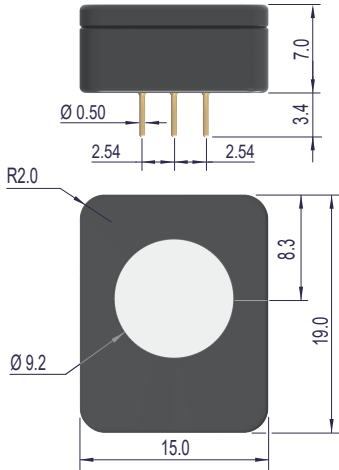
所有尺寸标注以毫米为单位 除非另有说明, 所有公差±0.20毫米
