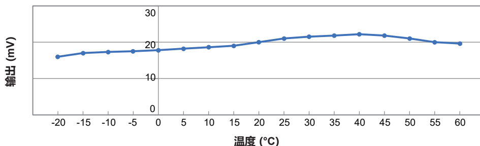
环境温度影响 (在1%甲烷中)
